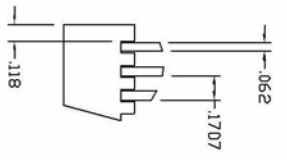
FIN DETAIL
